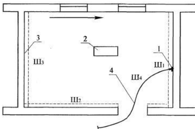
Рис.19. Схема организации рабочего места звена № 1
