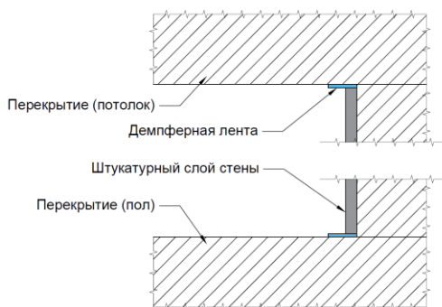
Рис.17. Приклейка демпферной ленты в местах сопряжения штукатурного слоя со стеной и потолком
