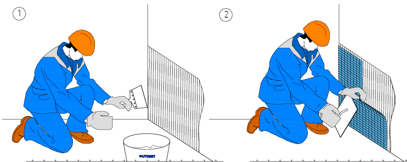
Рис. 25. Организация работ по приклеиванию мозаики
