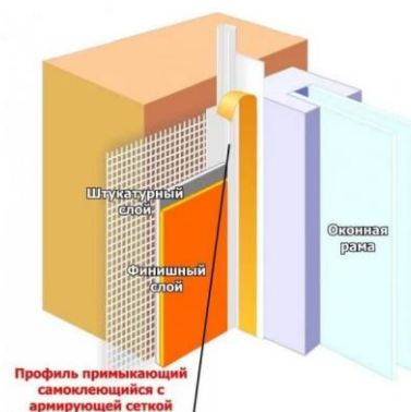
Рис.18. Профиль примыкающий с армирующей сеткой
